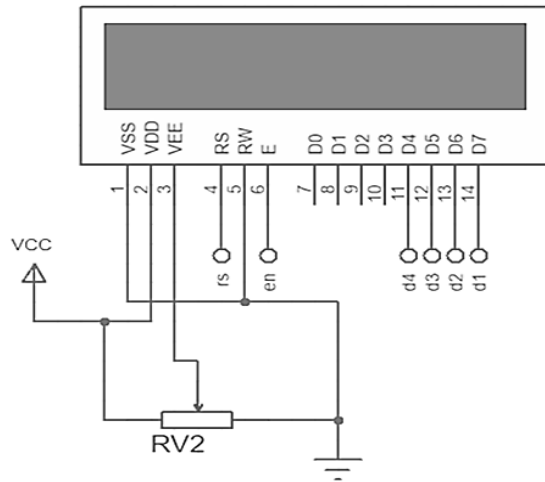
Fig. 4. LCD1 LMO16L unit (Ojha et al., 2016)
