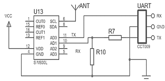
Fig. 5 SIM 800L unit (Waveshare, 2023)
